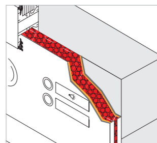
Isolierte Frontplatte
