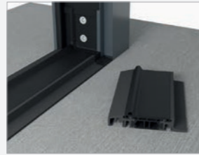
Bodenschwelle - Standard Schwarz, thermisch getrennt
